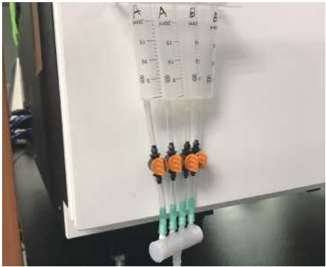
改善后：控制气体流量大小、流量可视
